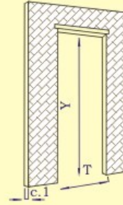
KAPI KASASINDA DUVAR BOŞLUĞU ÖLÇÜLERİ
