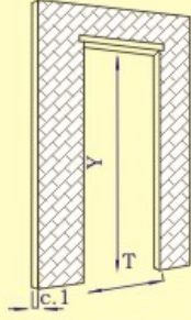
KAPI KASASINDA DUVAR BOŞLUĞU ÖLÇÜLERİ c: Duvar Kalınlığı Y: Duvar Boşluğu Yüksekliği T: Duvar Boşluğu Genişliği
