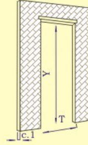
KAPI KASASINDA DUVAR BOŞLUĞU ÖLÇÜLERİ
