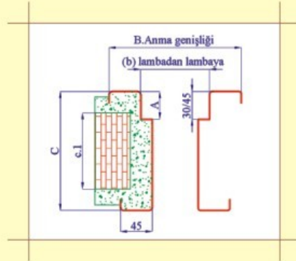
MONTE EDİLMİŞ KAPI KASASI ÖLÇÜLERİ H: Kapi Kasası Yüksekliği B: Kapi Kasası Genişliği
