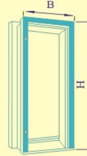
MONTE EDİLMİŞ KAPI KASASI ÖLÇÜLERİ H: Kapi Kasası Yüksekliği B: Kapi Kasası Genişliği
